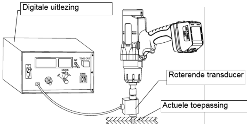
Test methode 3: dynamische meting met roterende transducer op de actuele toepassing.
