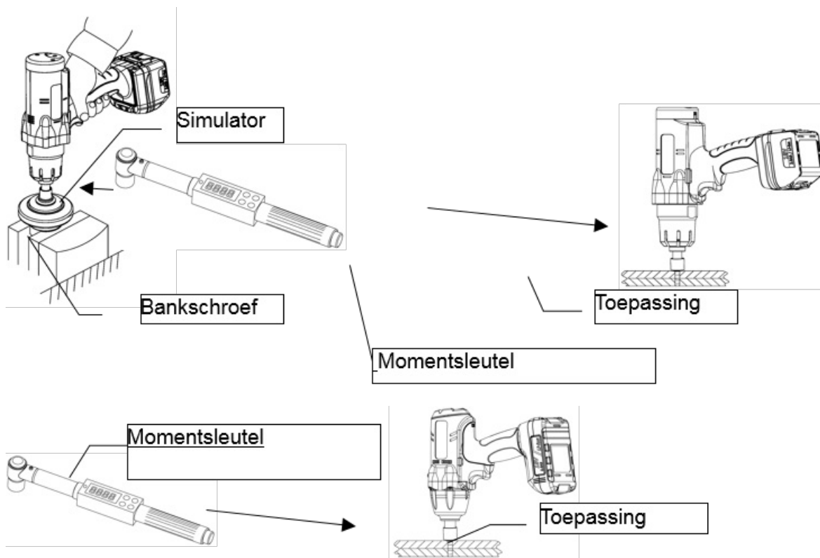
Test methode 2: dynamische meting met roterende transducer op een simulator.
