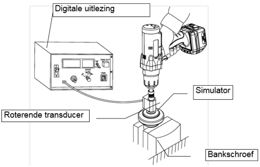
Test methode 3: dynamische meting met roterende transducer op de actuele toepassing.
