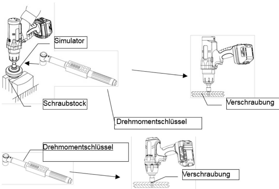
Messverfahren 2: dynamische Messung mit rotierendem Messwertaufnehmer auf einem Simulator.
