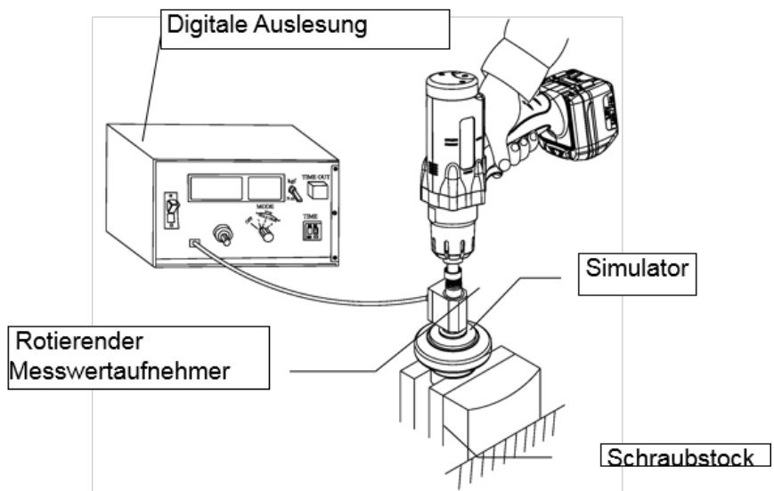
Messverfahren 3: dynamische Messung beim aktuellen Schraubfall.
